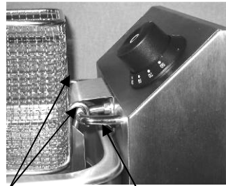
Haken Frittierkorb
